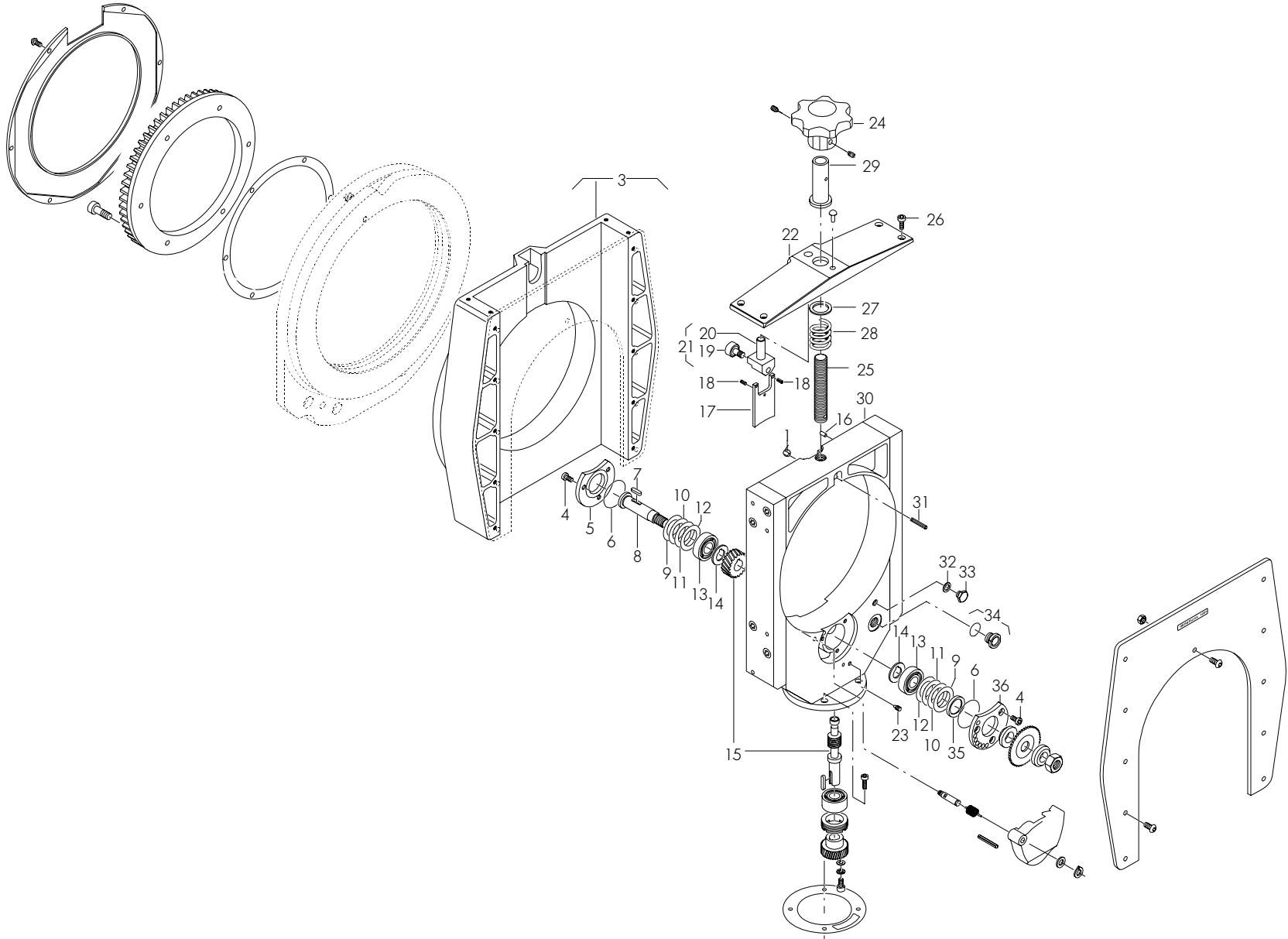
RA 8: Schieber, Drehkörper/Slide, revolute (Fig. 1)
